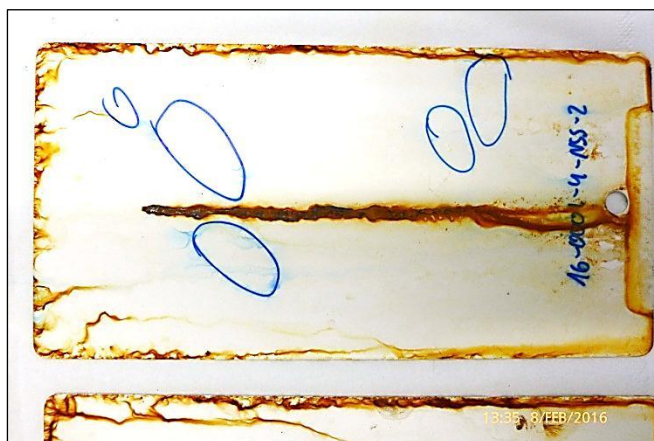
(a) Probeta "16-0001-4-2", aspecto general después de ensayo.
